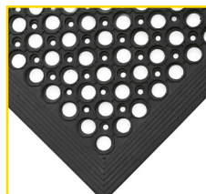
Surface alvéolaire
